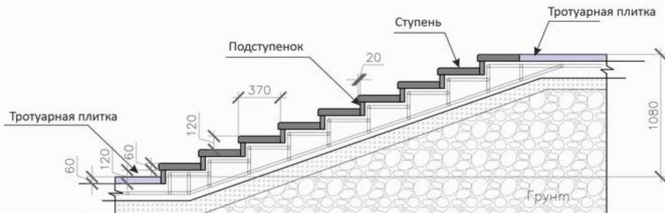
Разрез монтажа ступеней и подступенков
