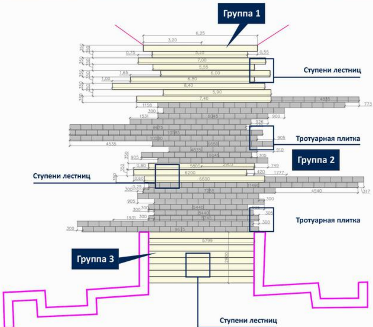
Схема раскладки из с альбома от архитектурного бюро г. Воронеж
