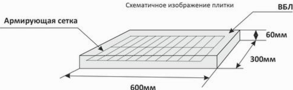
Схематичное изображение плитки
