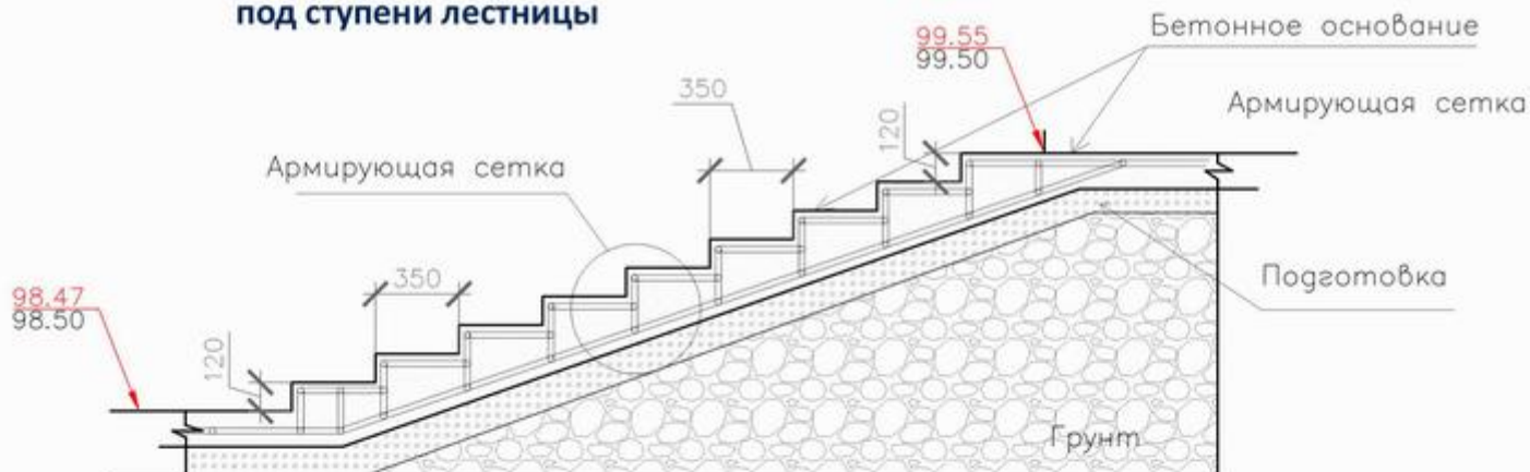
Группа ступеней 1 Схематичный разрез бетонного основания под ступени лестницы
