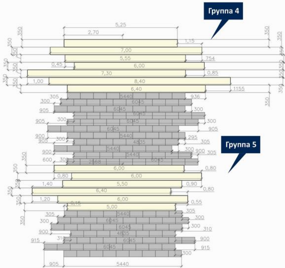
Группа ступеней 4 Раскладка
