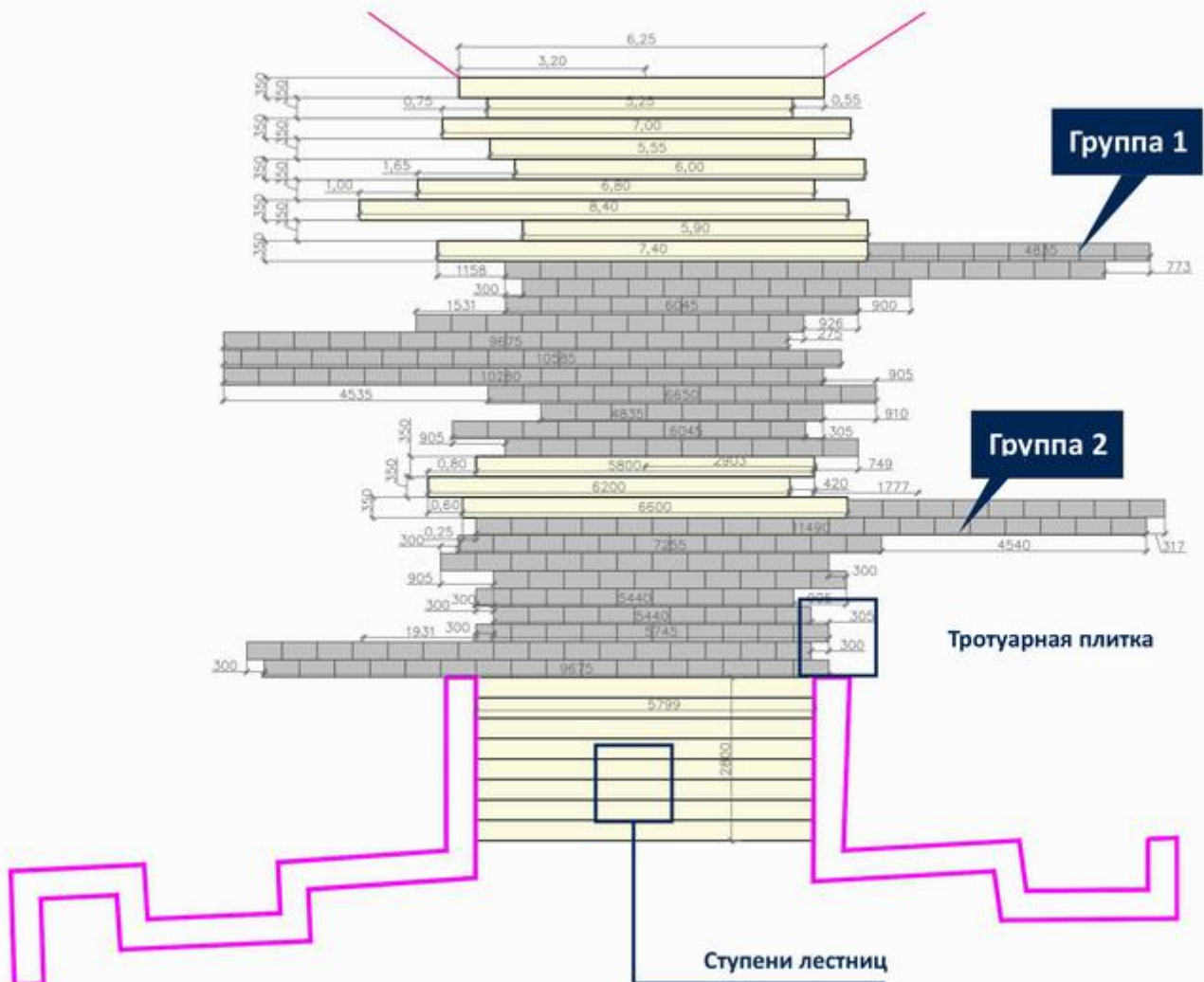
Схема раскладки из с альбома от архитектурного бюро г. Воронеж
